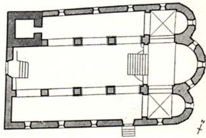
Spiez, Schlosskirche, Längsschnitt und Grundriss
